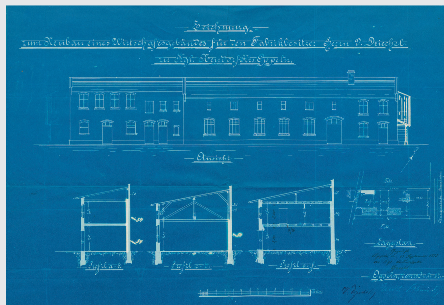
Rysunek techniczny pod budowę nowego budynku gospodarczego fabryki Dziechela w Nowej Wsi Królewskiej [Archiwum Państwowe w Opolu, sygn. 45/30/147]
